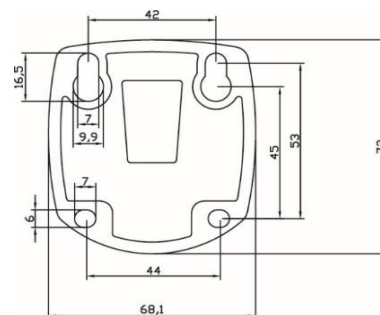
台座取付寸法
